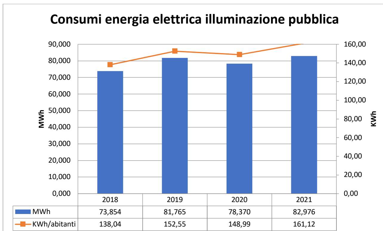
GRAFICO 9 CONSUMI ILLUMINAZIONE PUBBLICA FONTE: VALLECAMONICA SERVIZI E UFFICI COMUNALI
