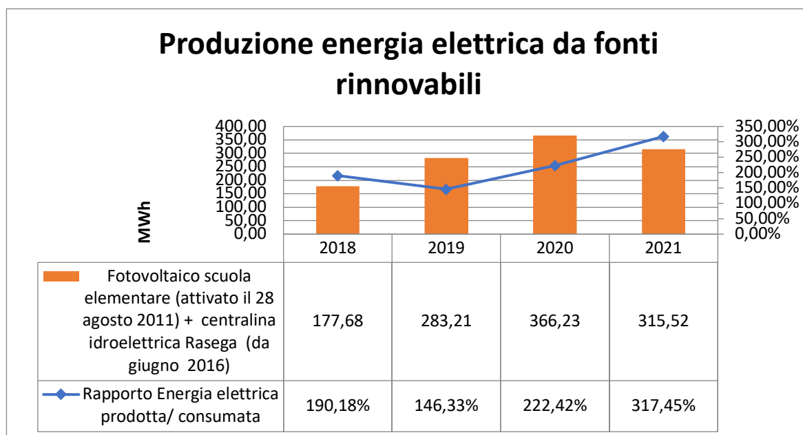
GRAFICO 7 RIEPILOGO PRODUZIONE ENERGIA ELETTRICA E RAPPORTO CON I CONSUMI DELL'ENTE
