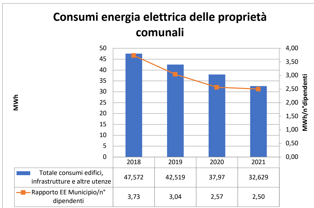
GRAFICO 8 CONSUMI DI ENERGIA ELETTRICA NEGLI EDIFICI COMUNALI
