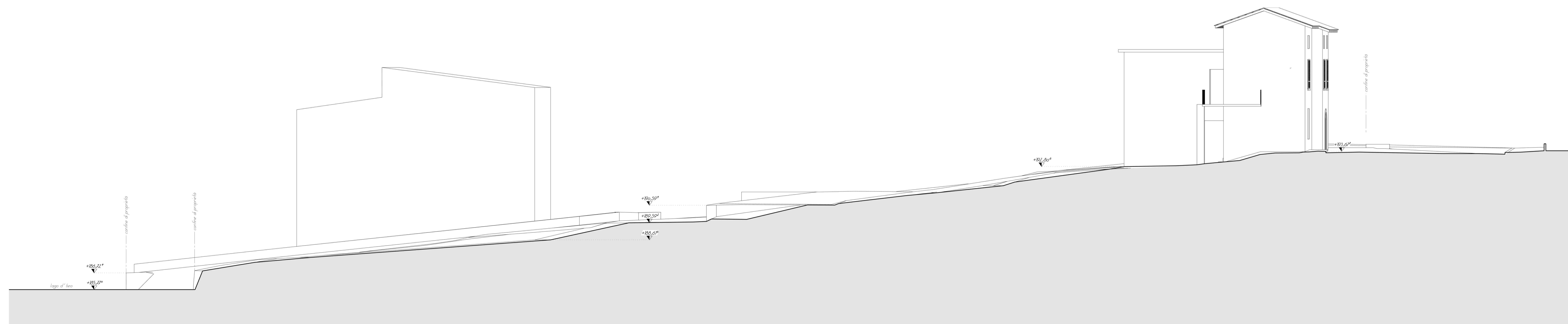
SEZIONE E-E - STATO DI FATTO - scala 1:100
