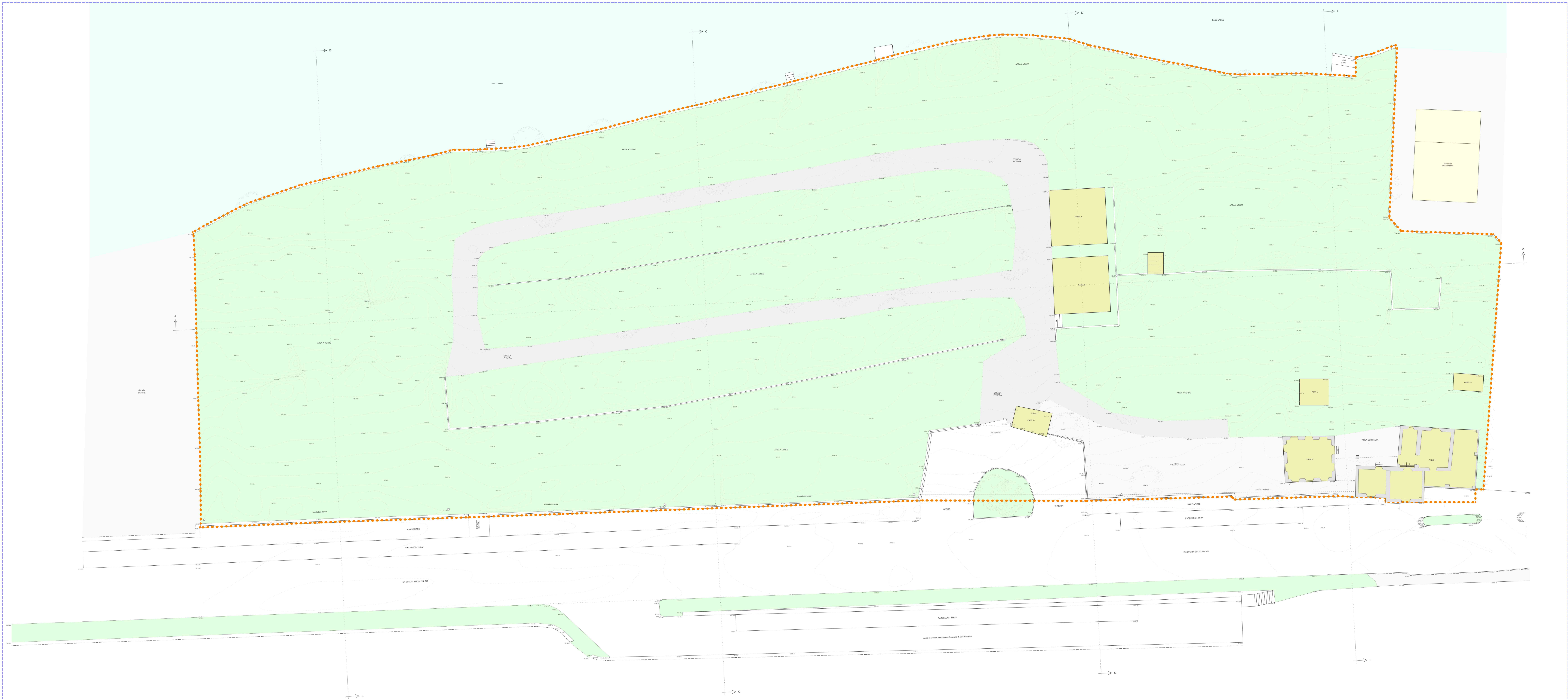
PLANIMETRIA GENERALE - STATO ATTUALE - scala 1:200
