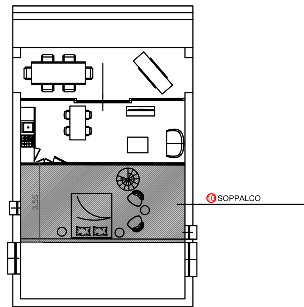
PIANTA COTTAGE CON SOPPALCO SCALA 1:100
