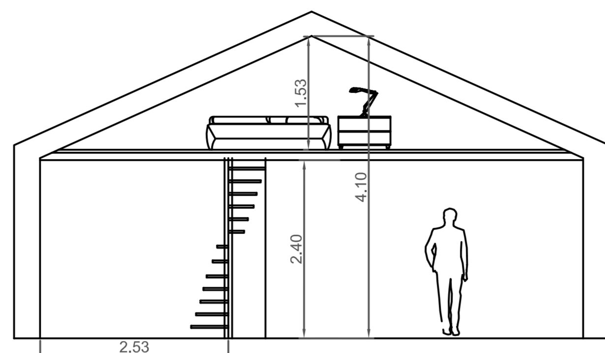
SEZIONE SOPPALCO SCALA 1:50
