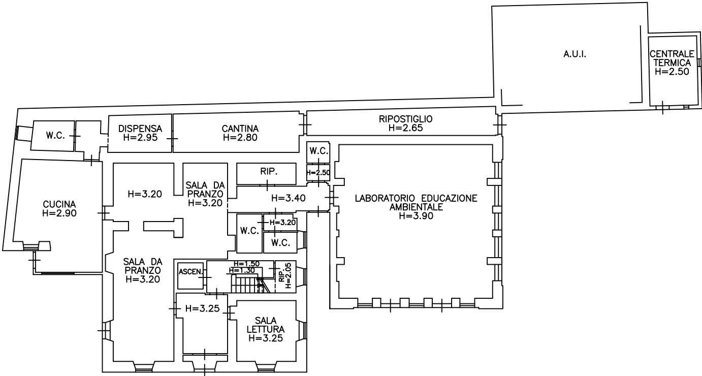
PIANTA P. SEMINTERRATO (S1)
