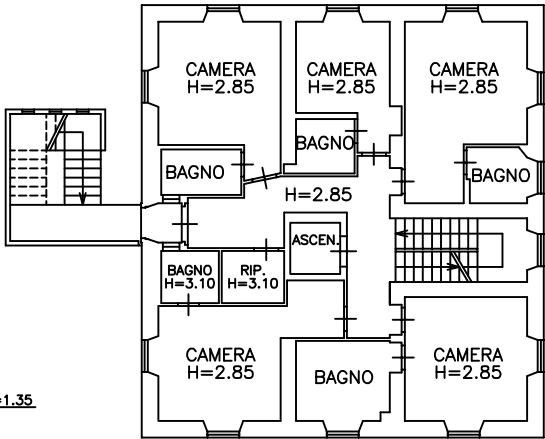
PIANTA P. SECONDO
