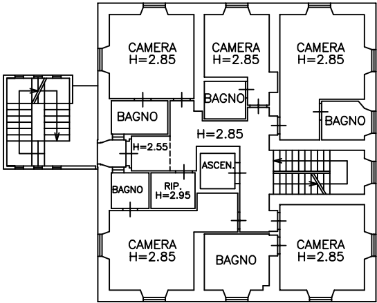
PIANTA P. PRIMO
