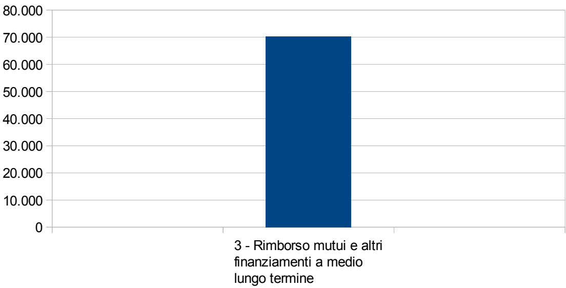
Diagramma 13: Indebitamento
