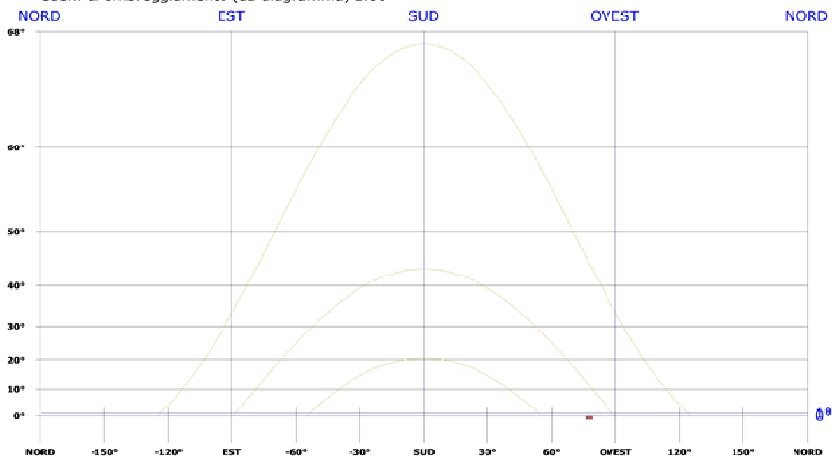
Fig. 2: Diagramma solare
