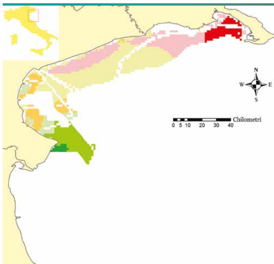
Figura 7.36 Risultato del modello spaziale per la valutazione dell'idoneità delle aree per la mitilicoltura Fonte UNIMAR e ISPRA
