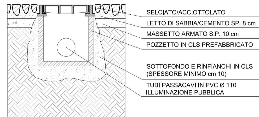
PARTICOLARE ISPEZIONE POZZETTO SCALA 1:20
