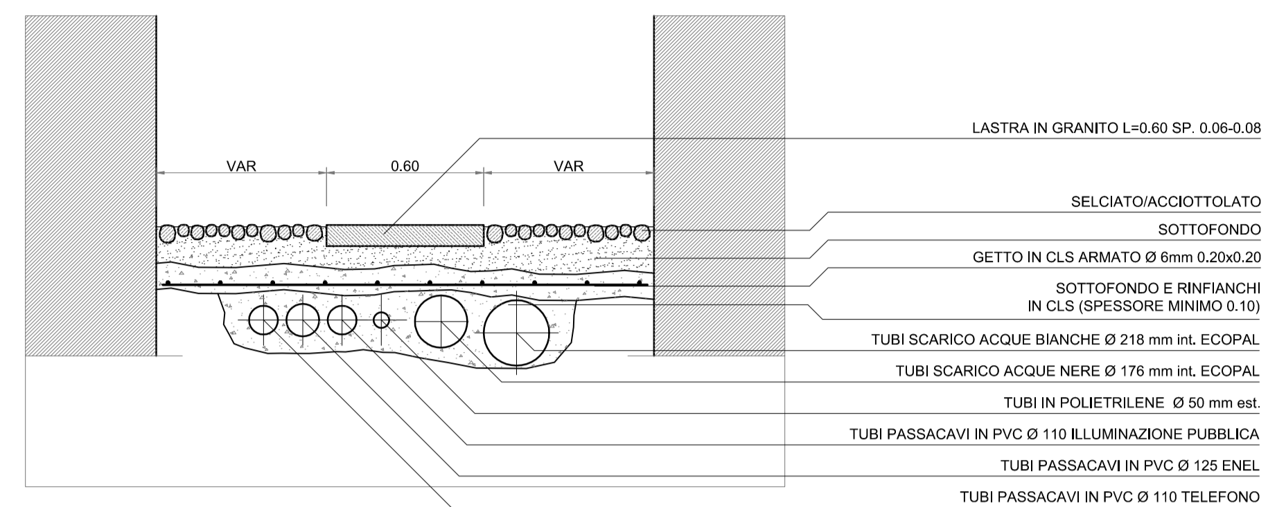
SEZIONE IN VIA CASTELLO SCALA 1:20
