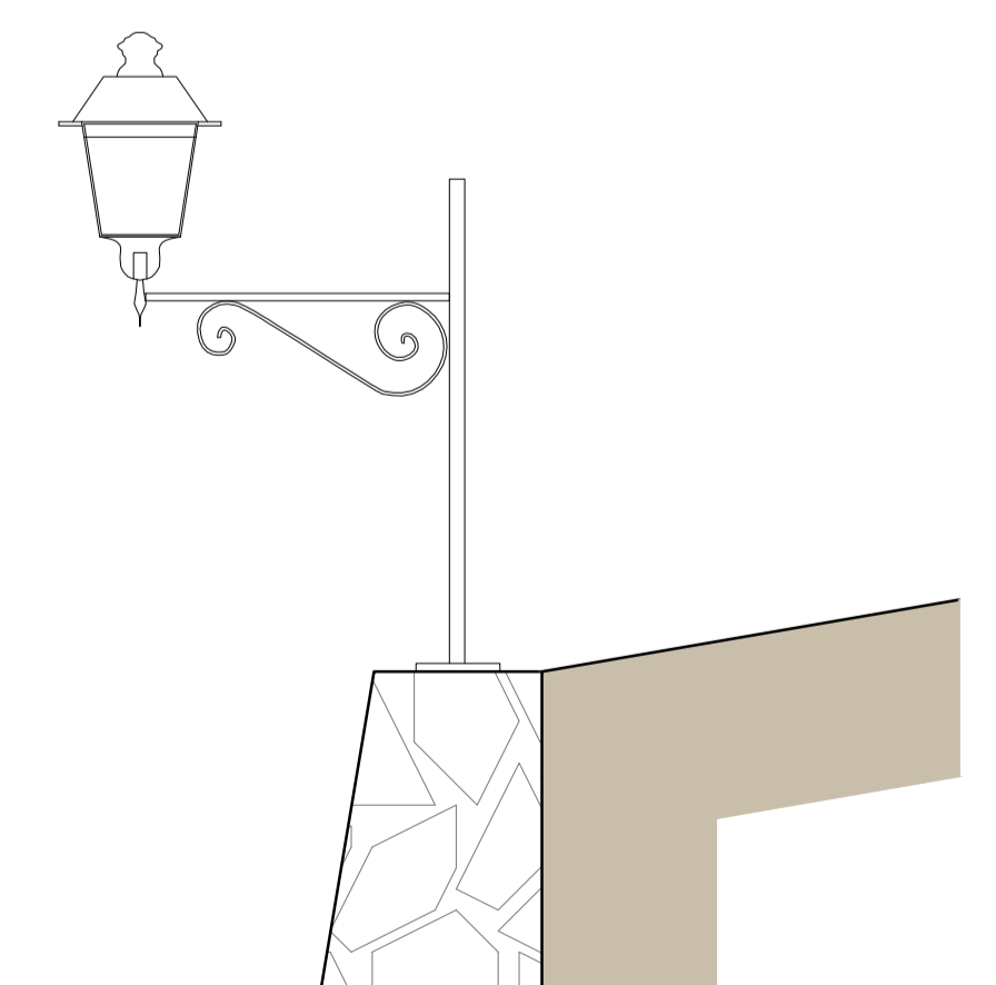
PARTICOLARE PUNTO LUCE ILLUMINAZIONE CON PALO
