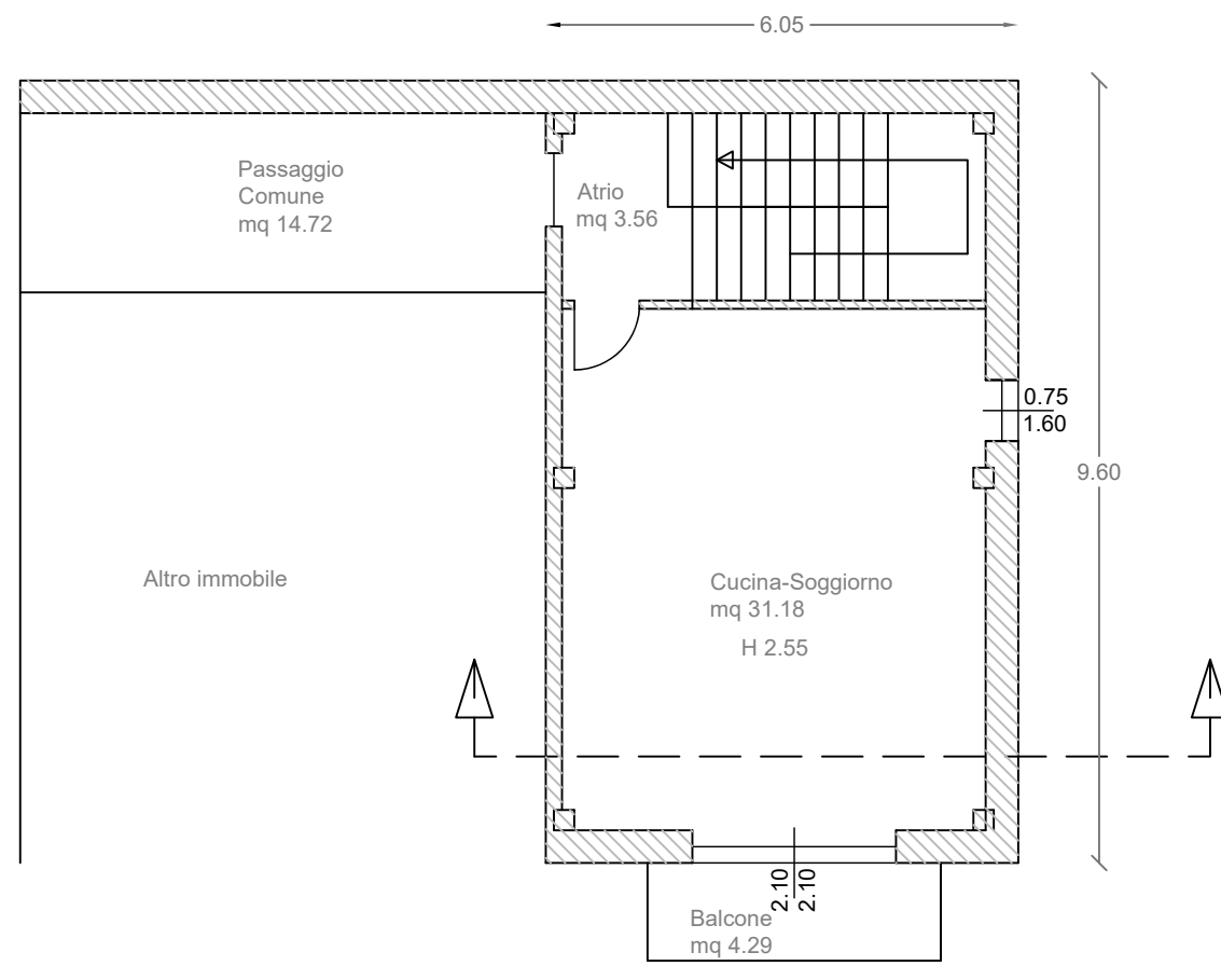
Immobile D Piano Rialzato Progetto
