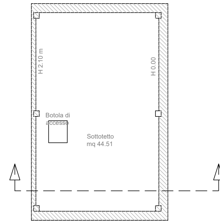
Immobile D Piano Sottotetto Esistente Invariato
