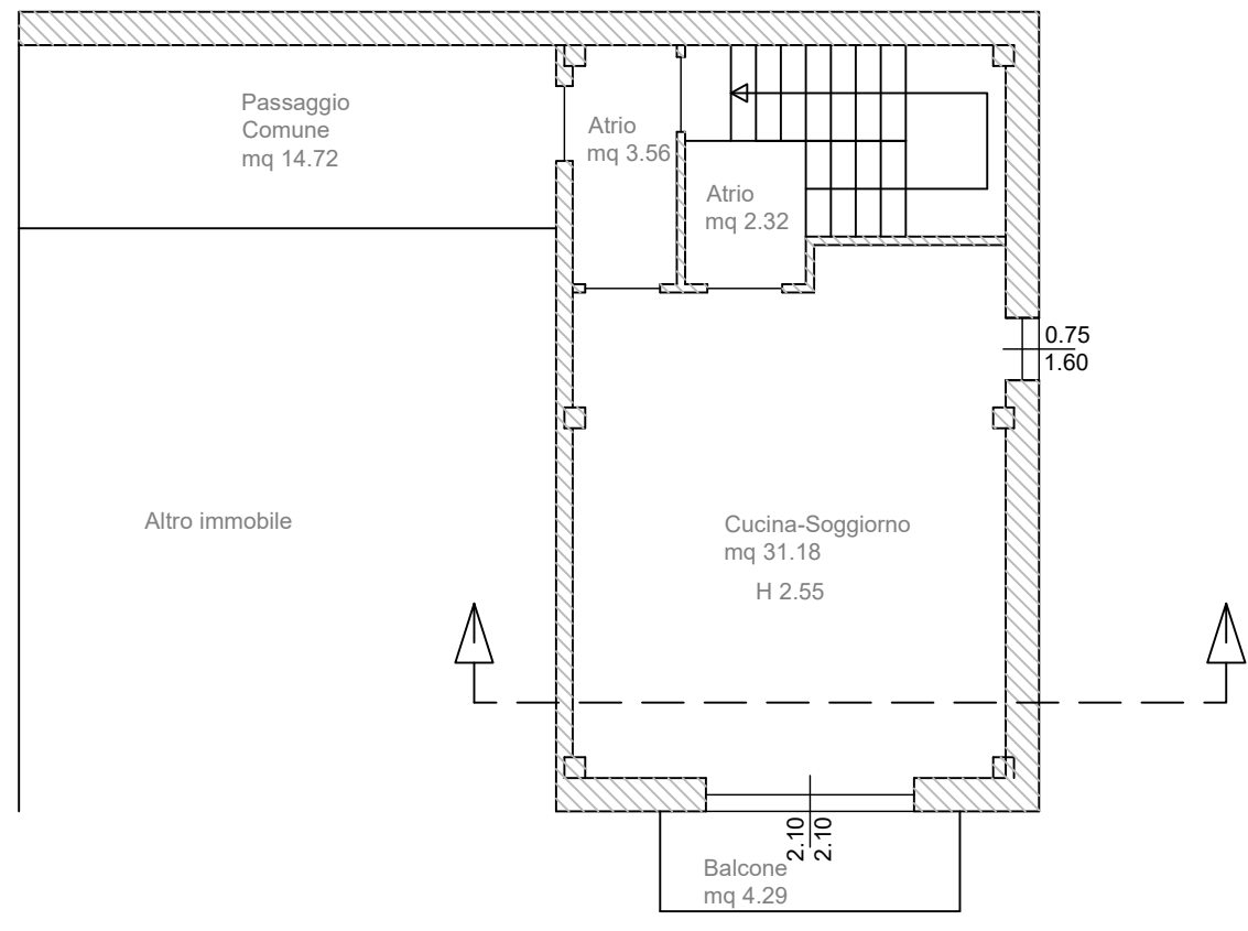
Immobile D Piano Rialzato Esistente
