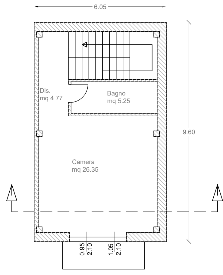
Immobile D Piano Primo Progetto
