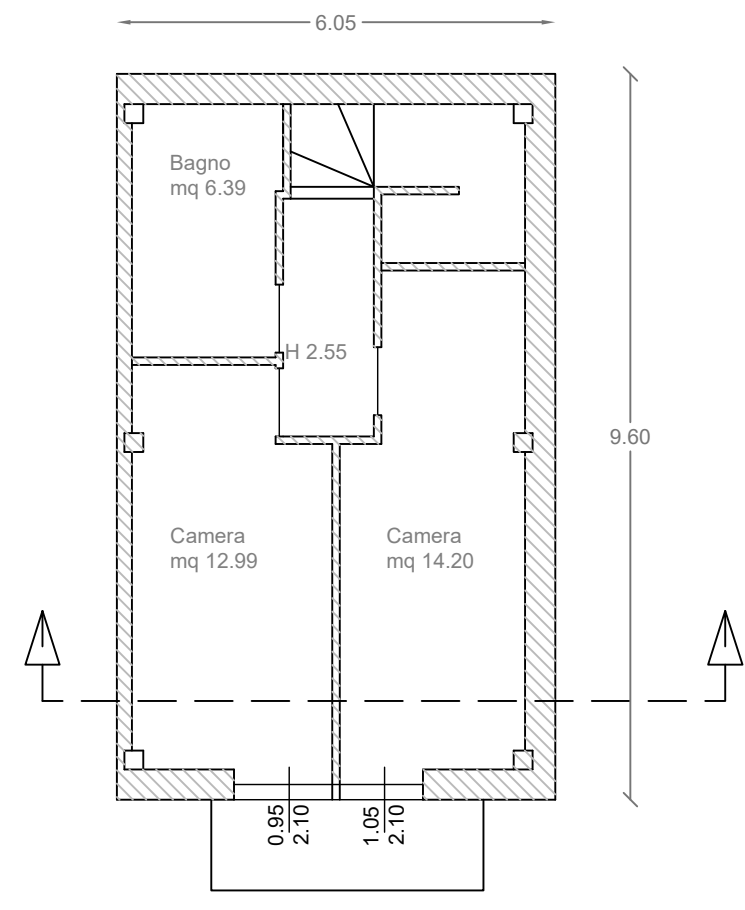
Immobile D Piano Primo Esistente
