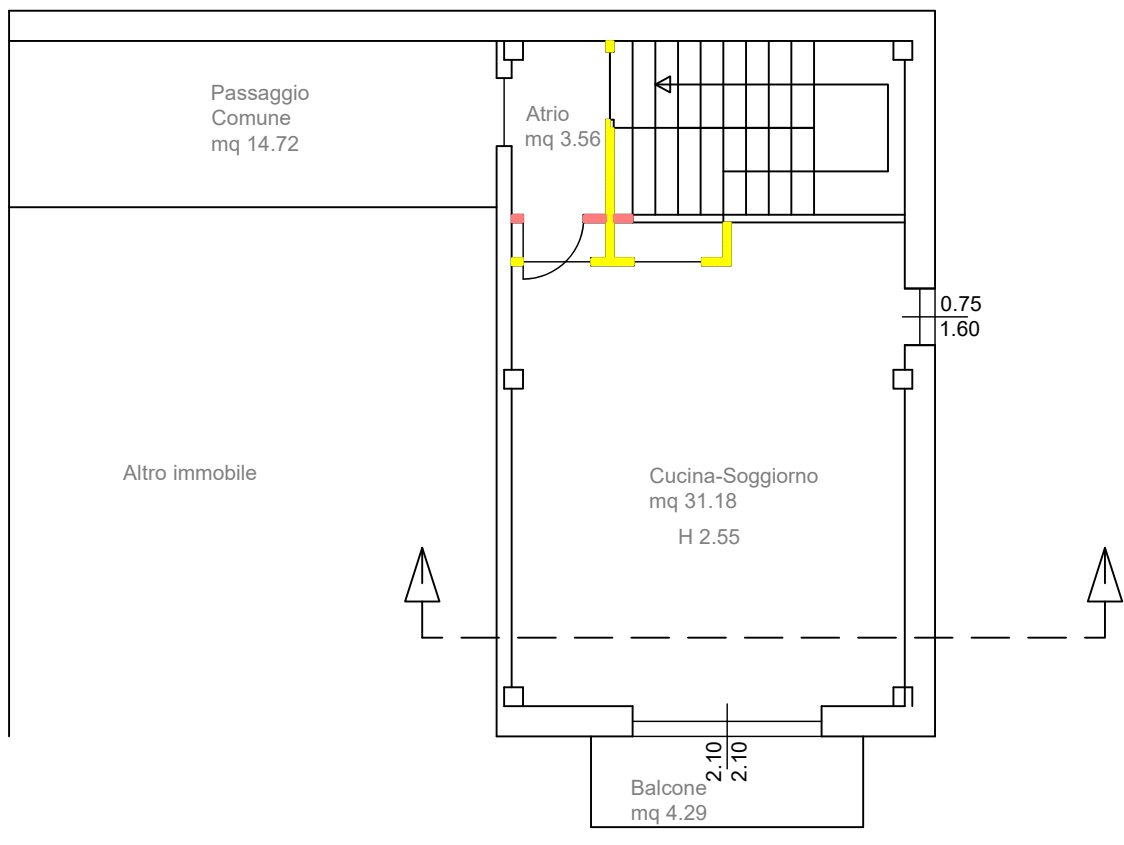
Immobile D Piano Rialzato Comparativo
