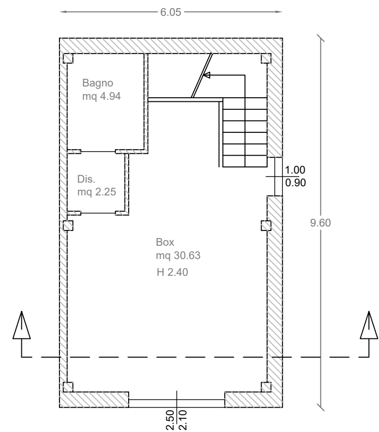
Immobile D Piano Terra Esistente
