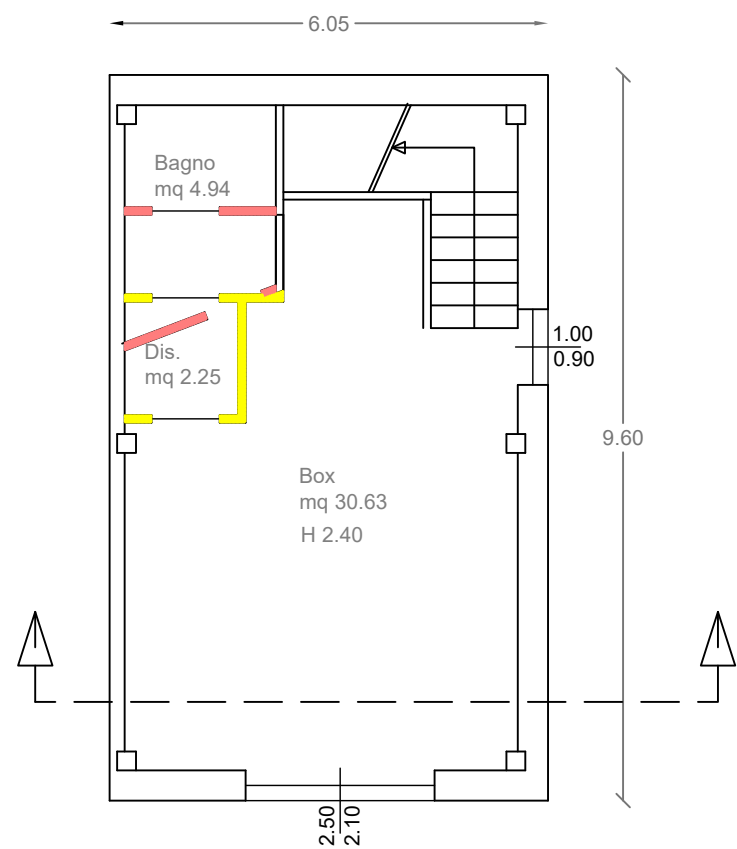
Immobile D Piano Terra Comparativo
