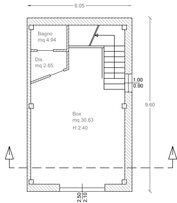
Immobile D Piano Terra Progetto
