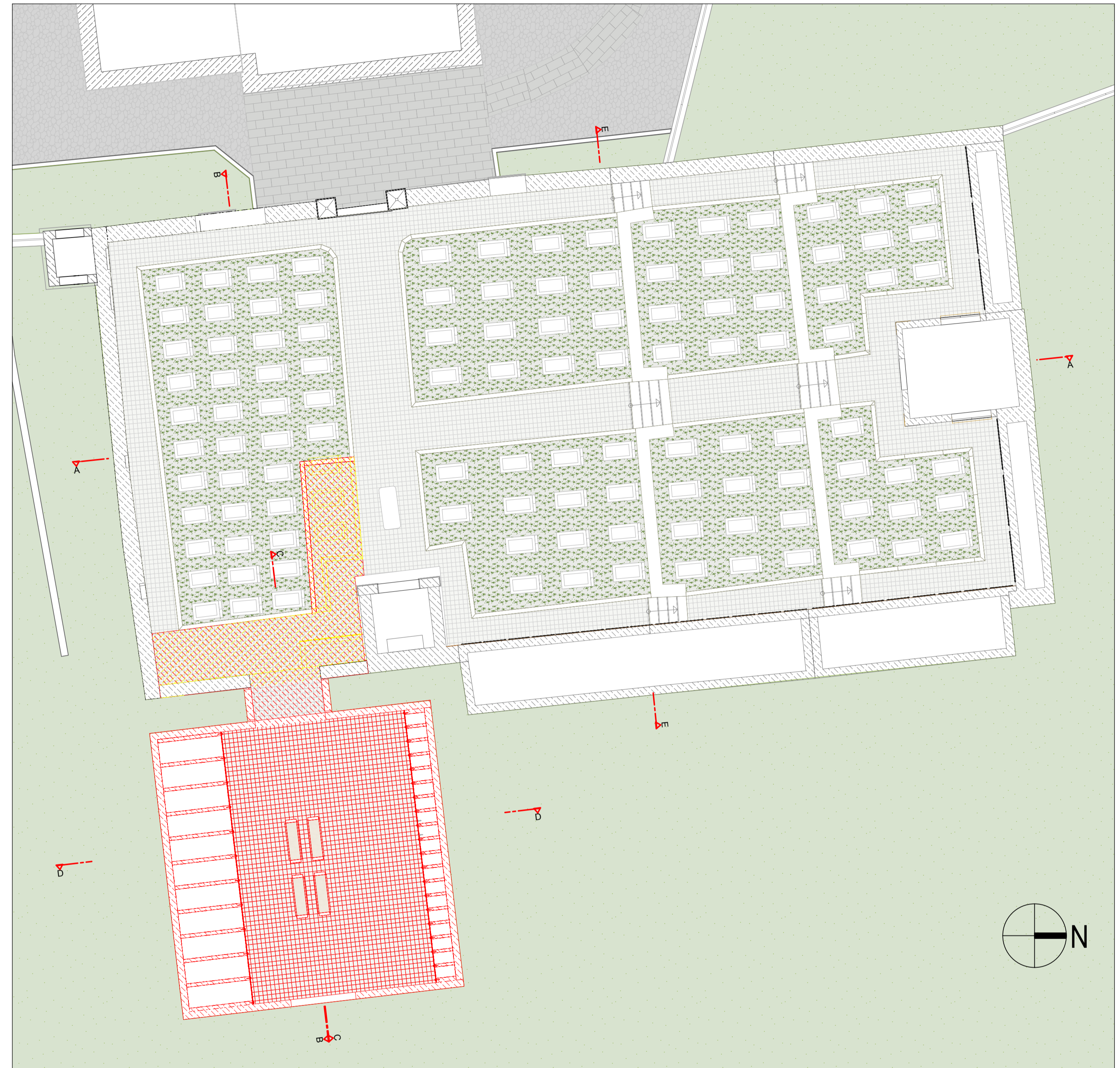
PIANTA DI RAFFRONTO - Scala 1:100
