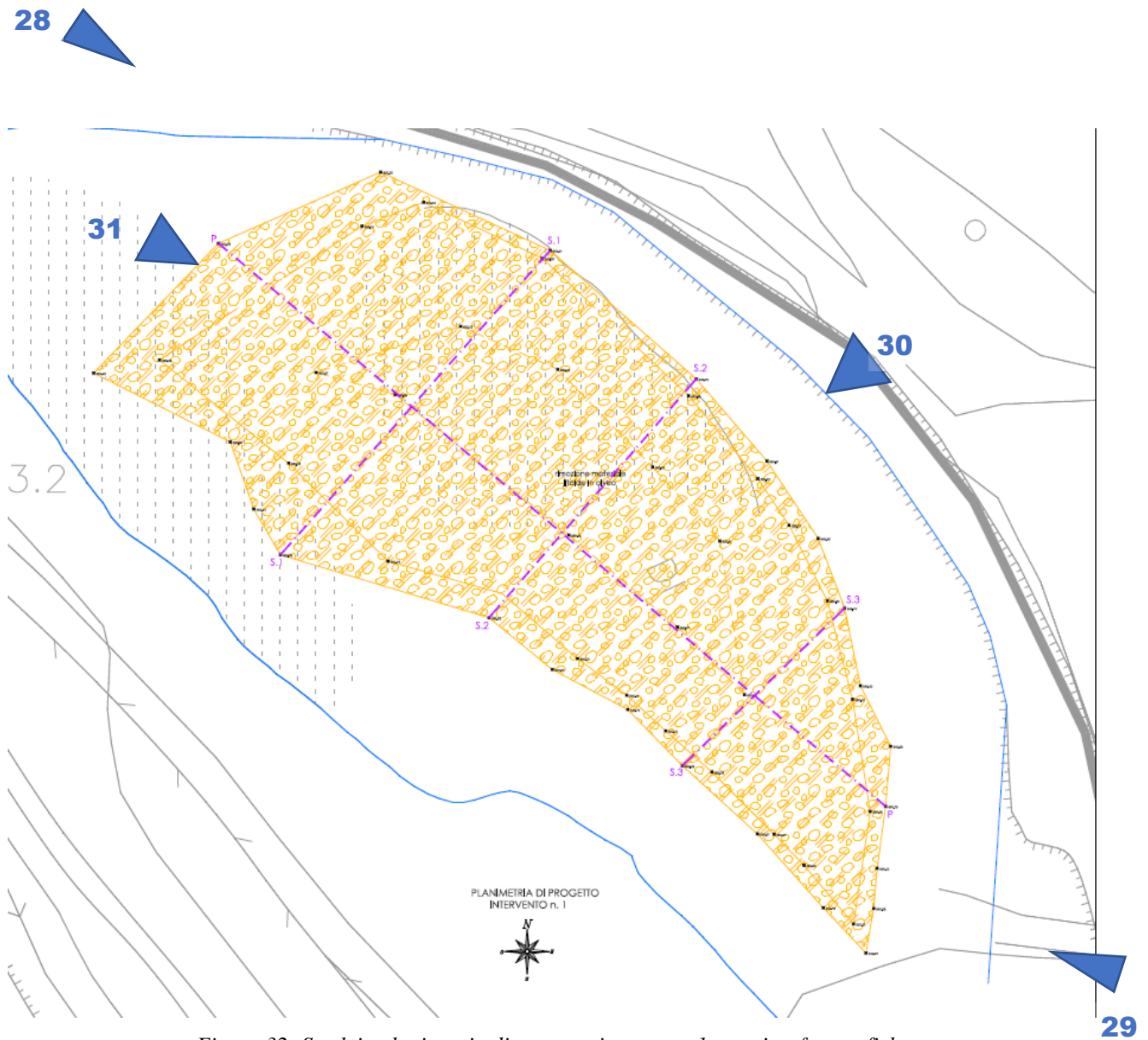
Figura 32: Stralcio planimetria di progetto intervento 1 con viste fotografiche
