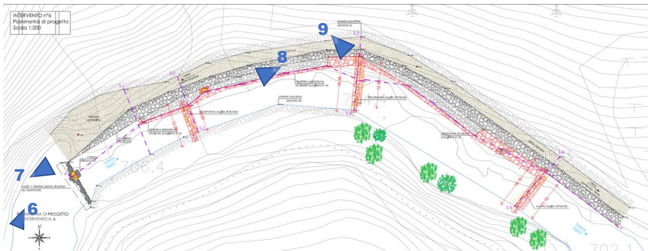
Figura 10: Stralcio planimetria di progetto intervento 6 con viste fotografiche
