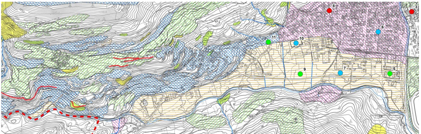
Figura 34: Stralcio Carta della Pericolosità Sismica Locale
