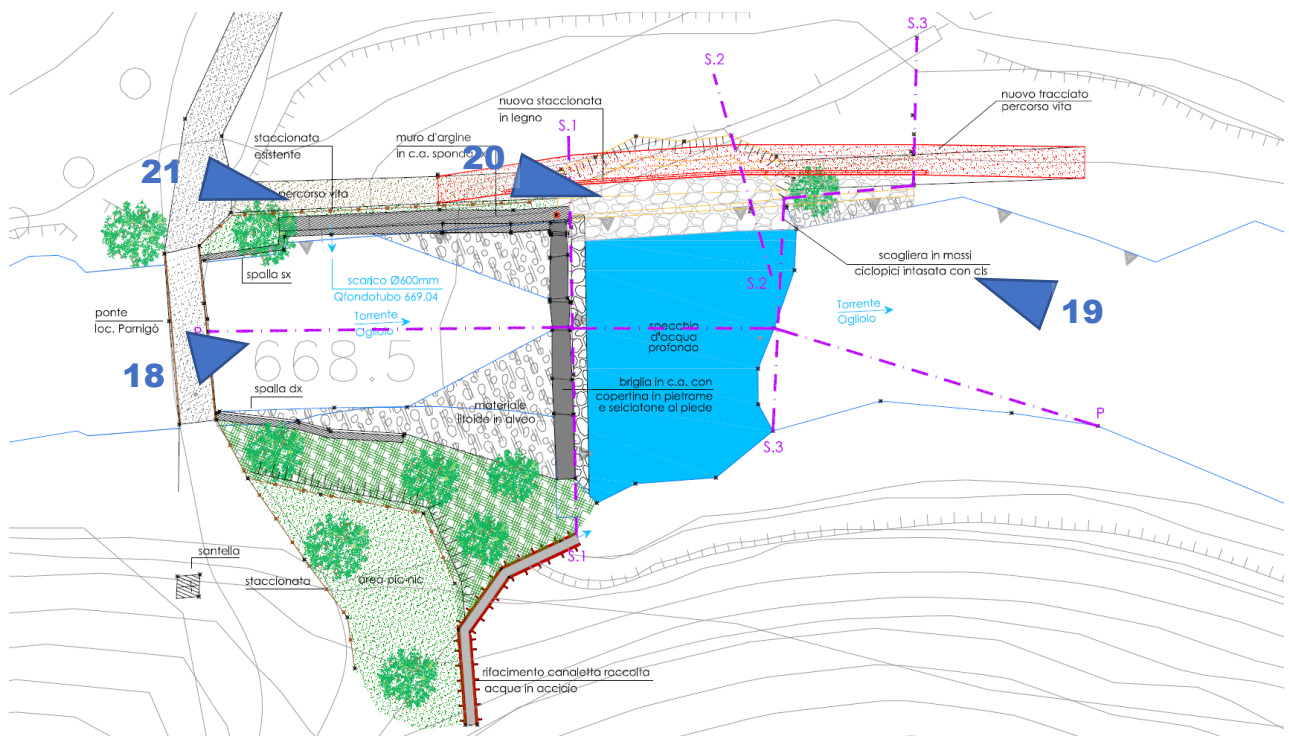
Figura 22: Stralcio planimetria di progetto intervento 3 con viste fotografiche
