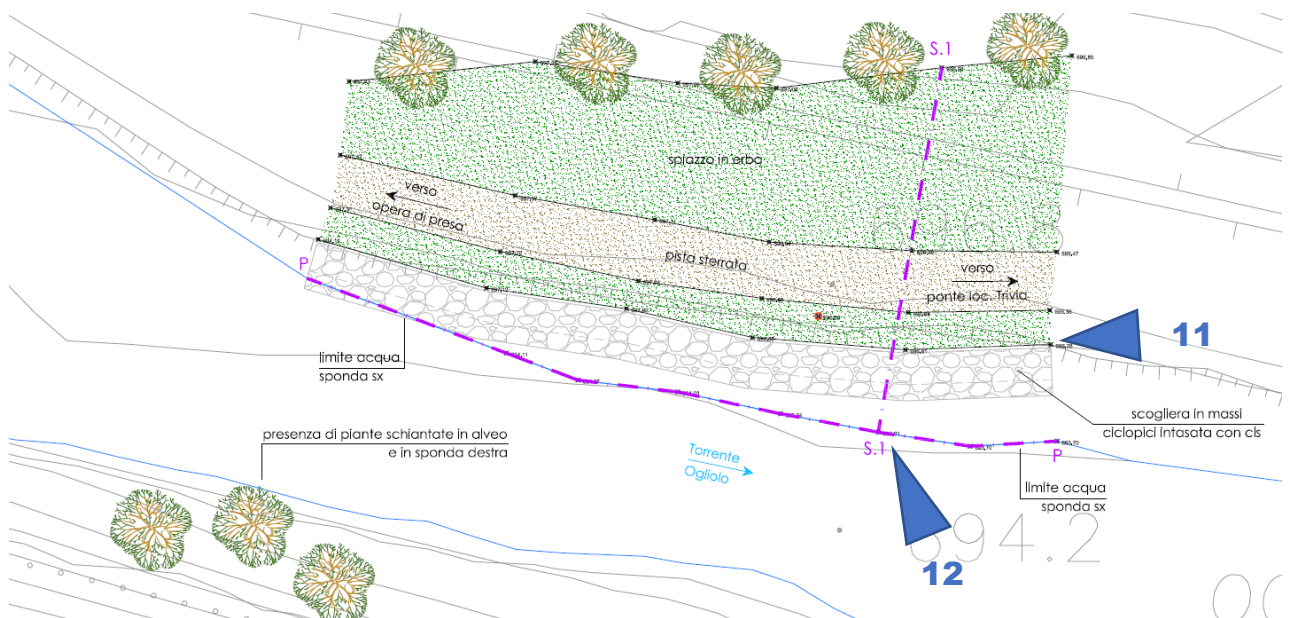
Figura 13: Stralcio planimetria di progetto intervento 5 con viste fotografiche
