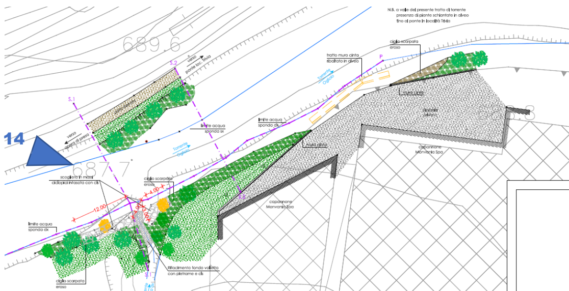
Figura 16: Stralcio planimetria di progetto intervento 4 con viste fotografiche
